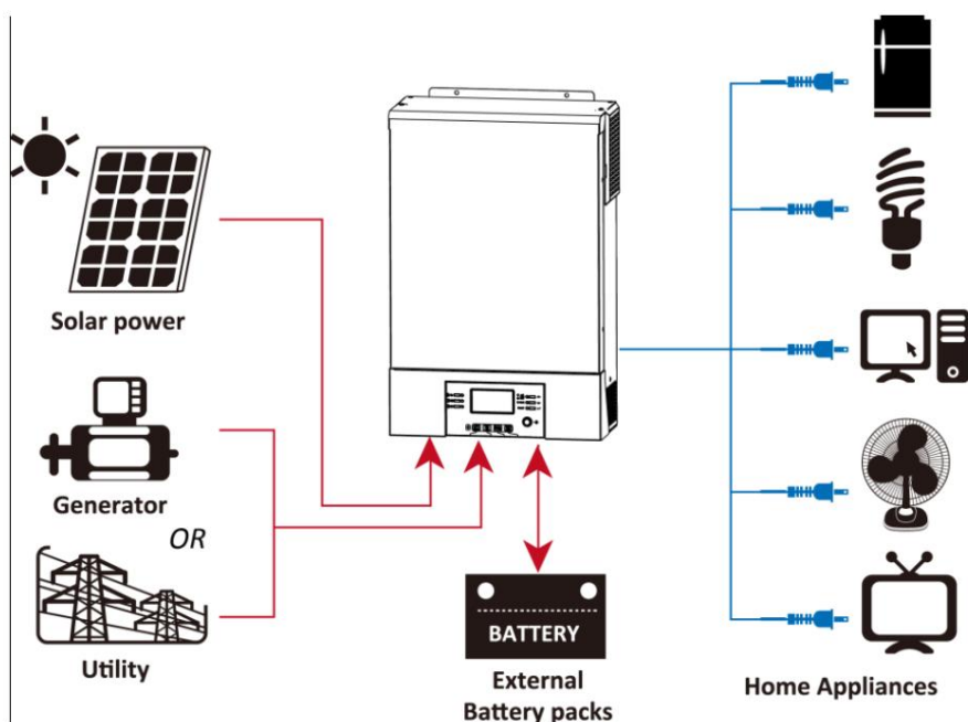
Obrázek 1 Hybridní energetický systém
